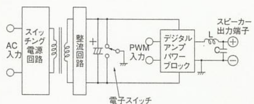
第4図 フローティング電源の原理図
