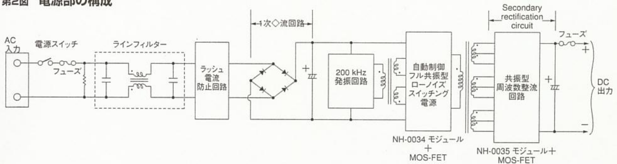
第2図 電源部の構成
