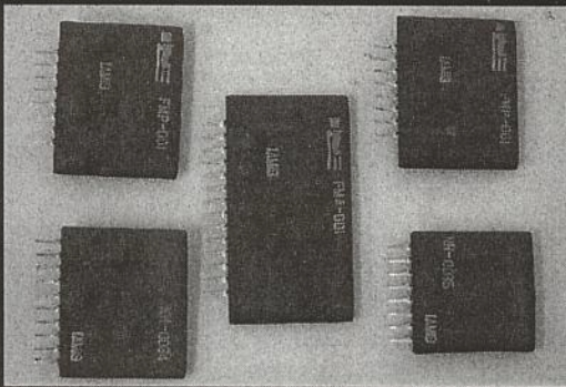
上段左右2個がFMP-001モジュール。中央がFMA-001モジュール、下段左がNH-0034モジュールで、下段右がNH-0035モジュール
