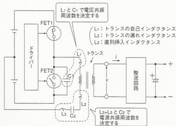
第3図 フルスイッチング電源の原理図
